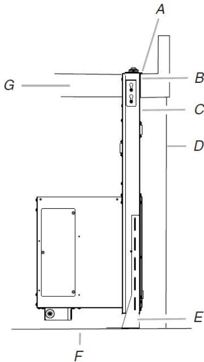
A. Lado trasero de ventilación retráctil B. Borde del corte en la cubierta C. Parte de atrás de ventilación retráctil D. Parte de atrás del gabinete E. Pata inferior de soporte F. Gabinete de piso G. Cubierta
