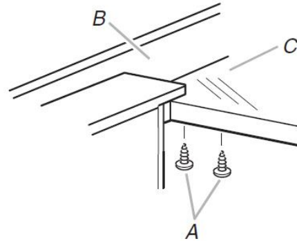
A. Tornillos B. Salpicadera C. Cubierta
