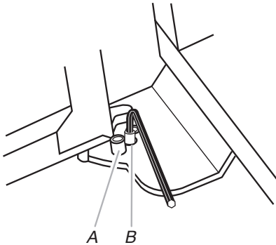
A. Tornillo del retén de la puerta de la parte inferior B. Tornillo del retén de la puerta de la parte superior (110°)
