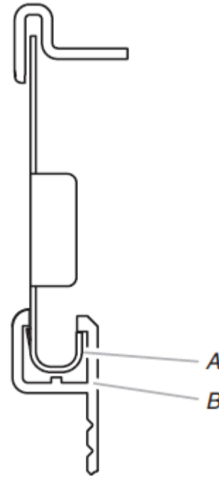
A. Rejilla de la base B. Faldón
